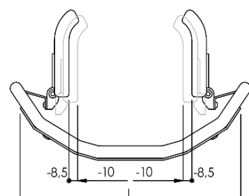
Support thoracique interne de la largeur du dossier, réglable (-8,5 ÷ -10cm)
