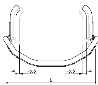
Support thoracique interne de la largeur du dossier, réglable (-4 ÷ -5,5cm)
